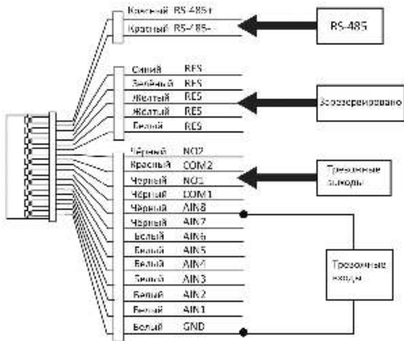
Рисунок 2-1-2 Распиновка коннектора ALARM/RS-485
