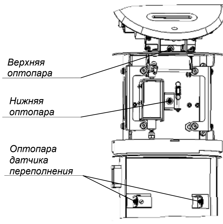
Рис. 3. Расположение оптопар картоприемника
