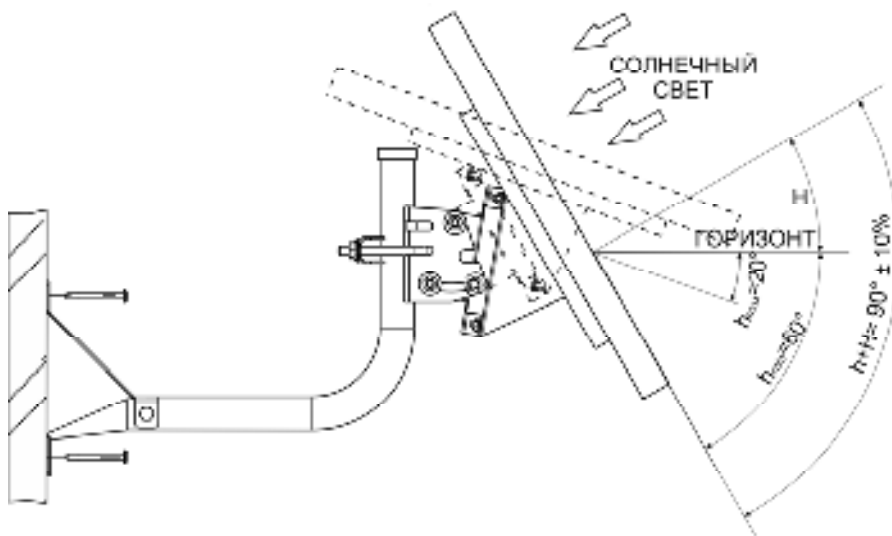
Рисунок 2 – установка изделия
