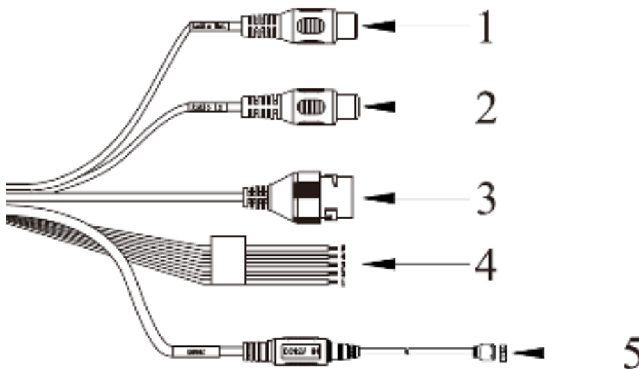
Рис. 2 Коммутационный кабель
