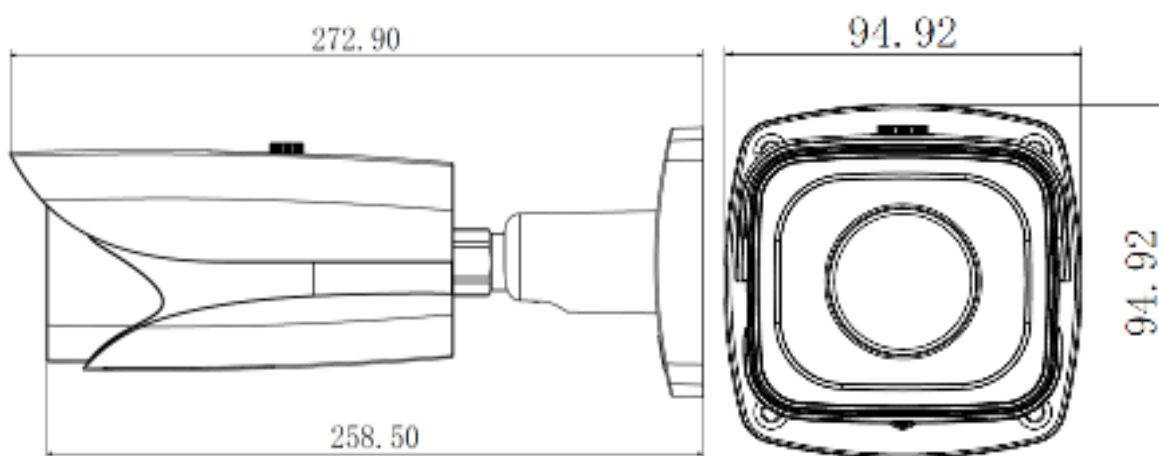
Рис. 1 Размеры камеры
