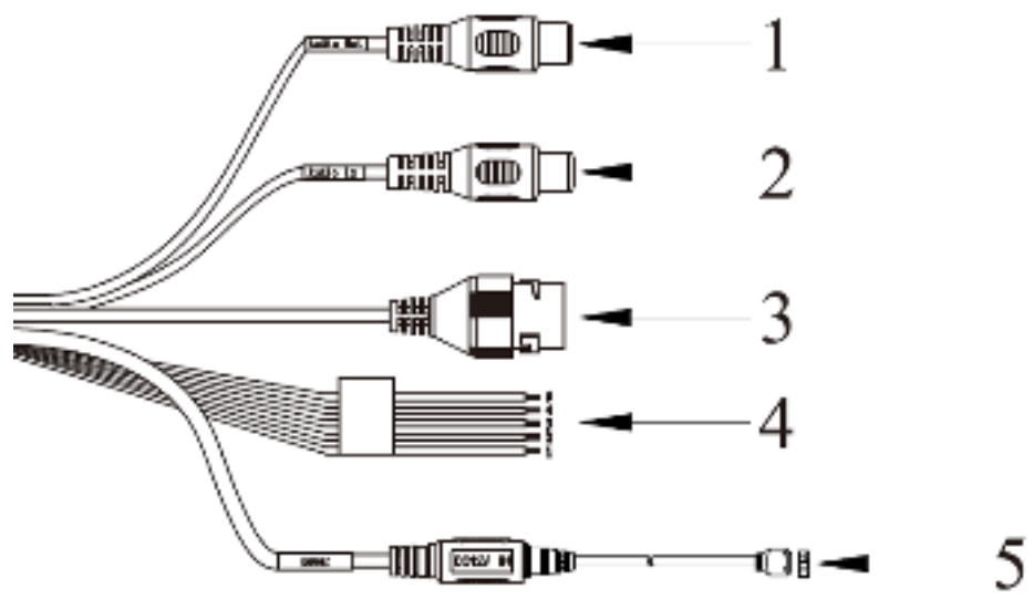
Рис. 2 Коммутационный кабель
