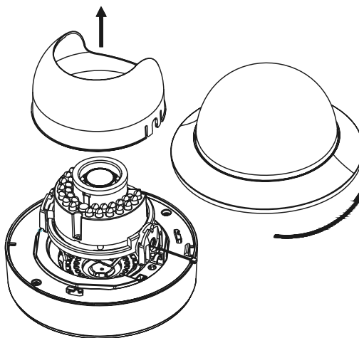
Рис. 2.1. Снятие купола с видеокамеры
