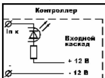
Рисунок 4 – Схема входных каскадов «In x»
