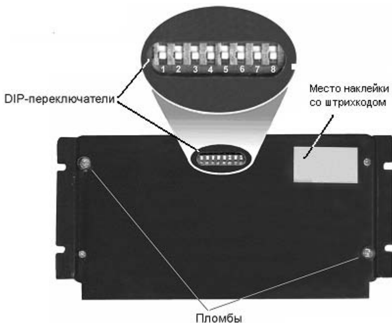
Рисунок 5 – DIP-переключатели контроллера
