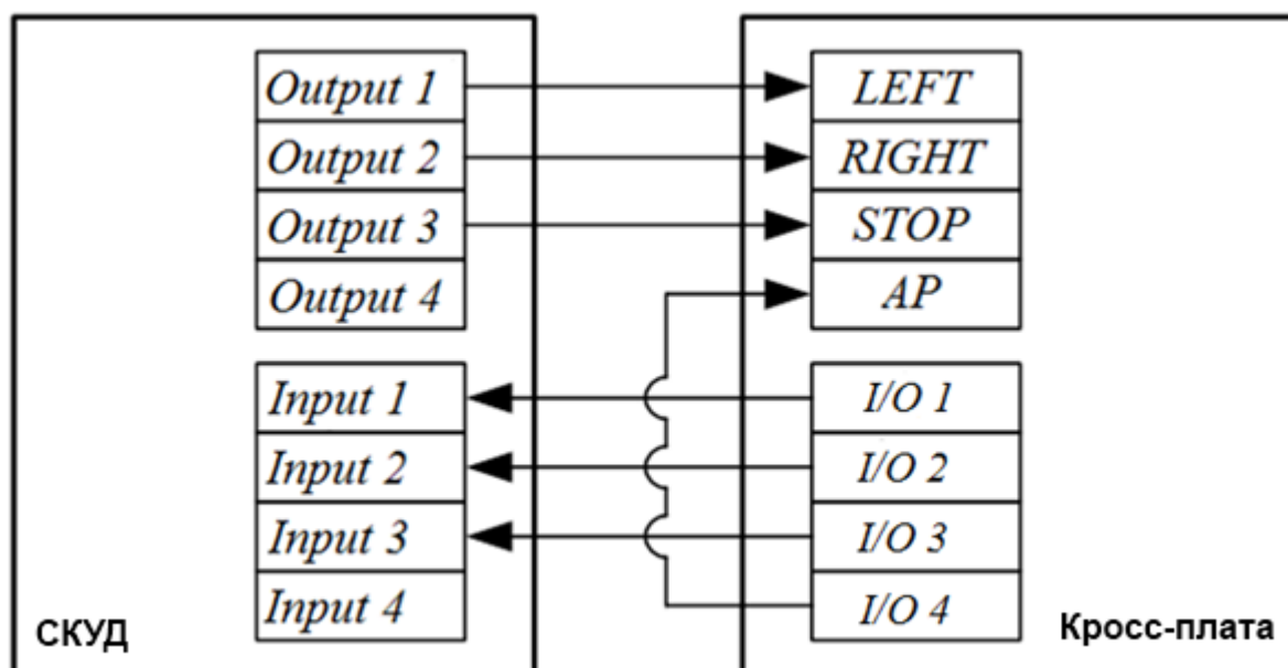
Рисунок 10 – Схема подключения ПУ к контроллеру СКУД
