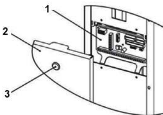
1 - кросс-плата; 2 - дверца стойки турникета; 3 - замок дверцы
