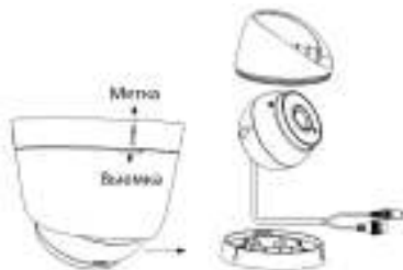
Рисунок 2-11 Демонтаж камеры
