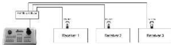
Подключение «звездой» с использованием распределителя сигнала RS-485
