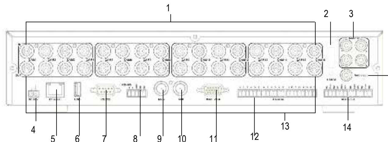
Рисунок 1-2 Задняя панель
