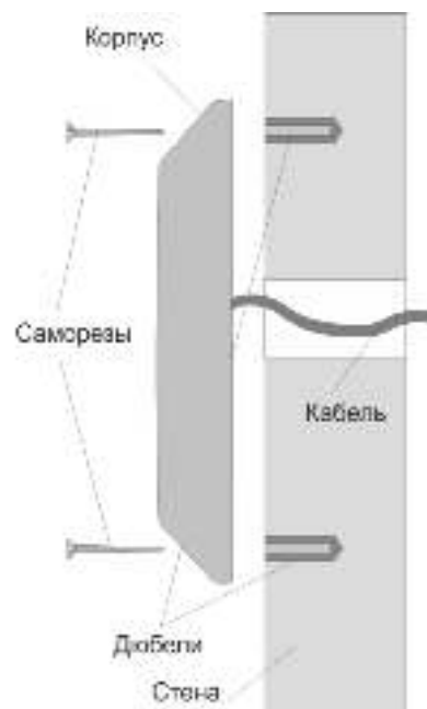
Рисунок 2. Крепление считывателя
