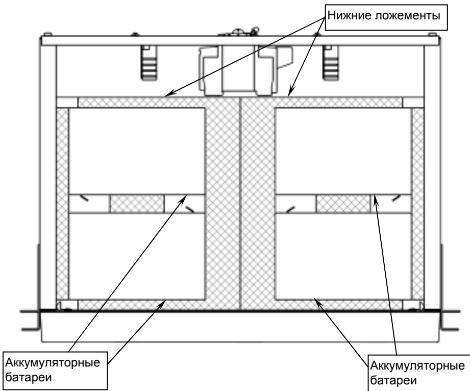
Рисунок 3 – Размещение аккумуляторных батарей в корпусе
