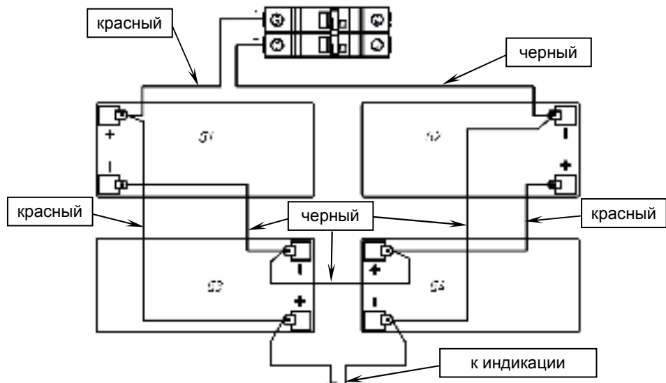
Рисунок 7 — Схема соединений аккумуляторных батарей
