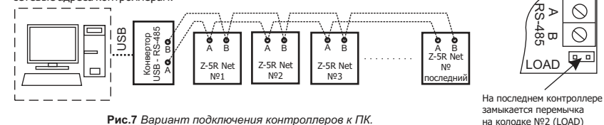
Рис.7 Вариант подключения контроллеров к ПК.
