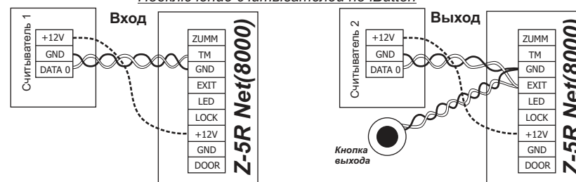
Рис 4. Подключение считывателей.
