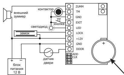
Рис 3. Подключение дополнительных элементов.
