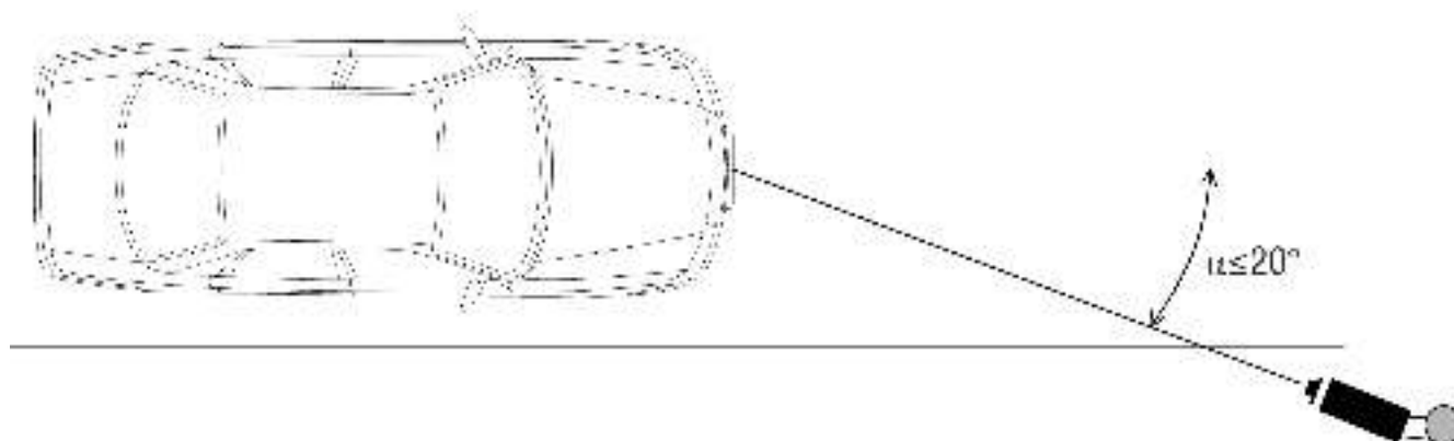
Рис. 4 Угол установки видеокамеры по горизонтали
