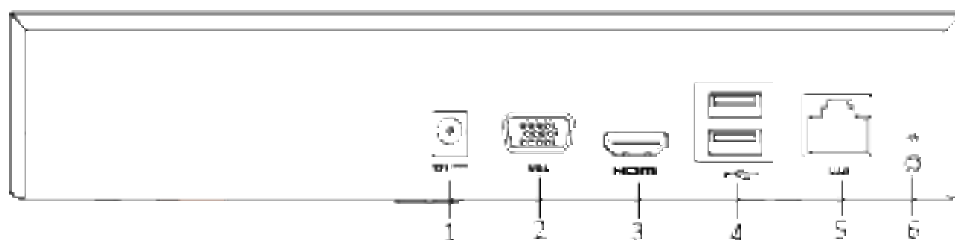
Рисунок 1.2 Задняя панель
