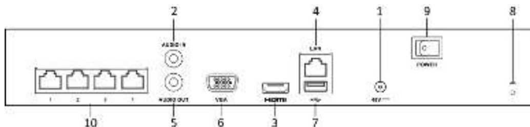
Рисунок 1.3 Задняя панель
