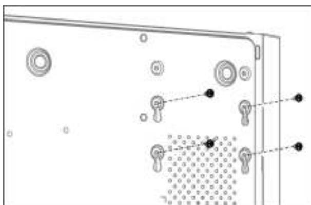
Рисунок 2.3 Фиксация HDD
