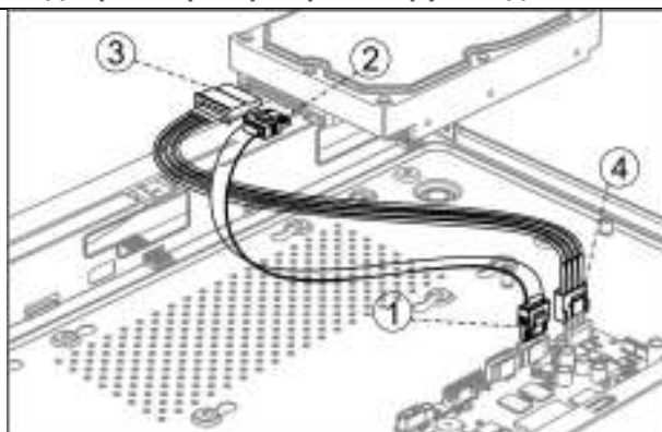
Рисунок 2.2 Подключение кабелей
