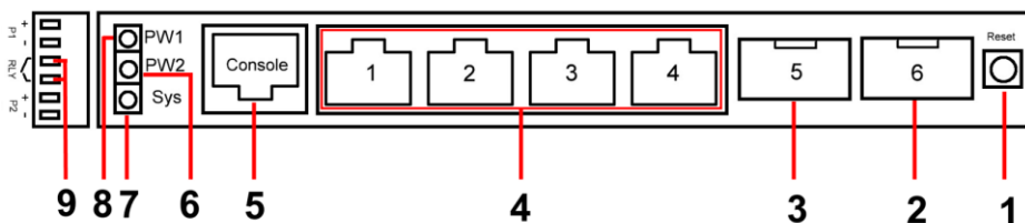
Рис.3 Уличный коммутатор SW-80402-WLU(port 90W), разъемы, кнопки и индикаторы
