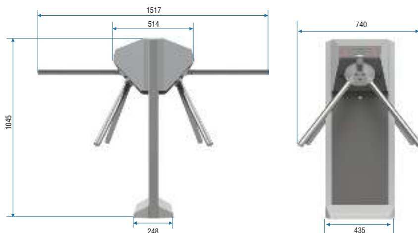
Рисунок 5.1 Габаритные размеры турникета «STL-04»
