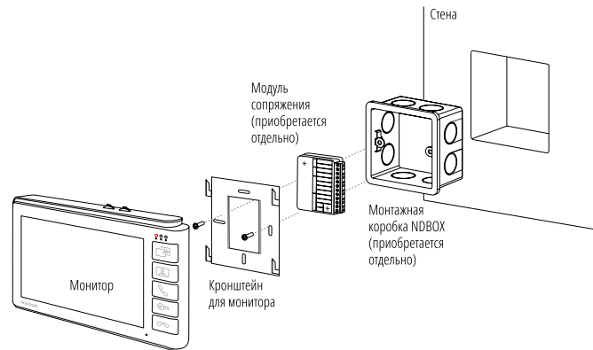
Рис. 6 Монтаж монитора SMILE 7 HD
