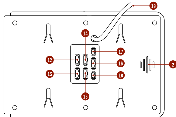
Рис. 3 Задняя панель монитора SMILE 7 HD
