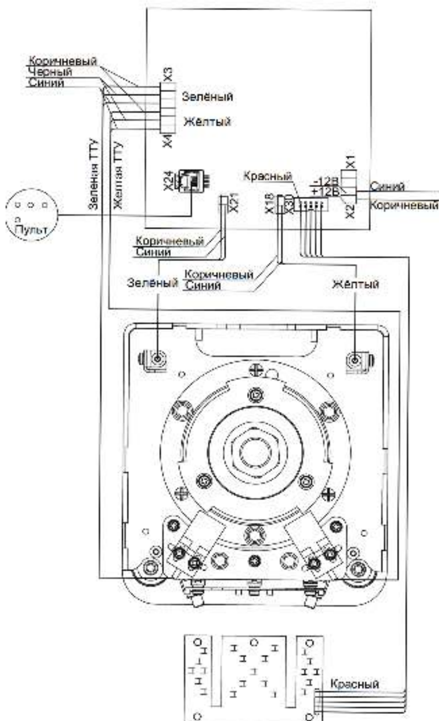
Рисунок 16 – Схема турникета
