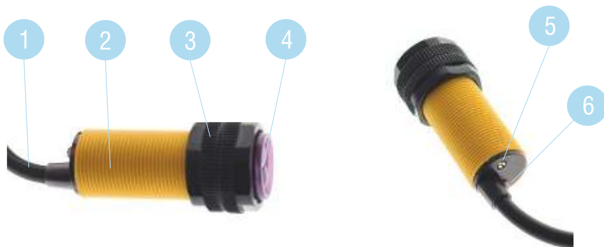
Рисунок 6.7.1 Устройство ИК-датчиков
