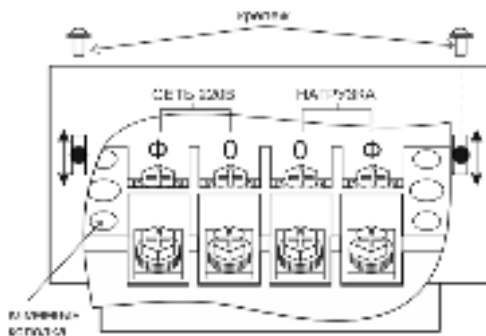
Рисунок 3 – Схема подключения к клеммной колодке
