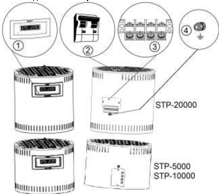
Рисунок 1 Общий вид стабилизатора и его функциональных элементов
