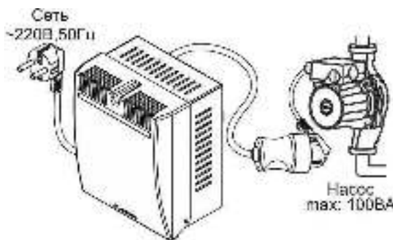
Рисунок 3 – Схема подключения изделия
