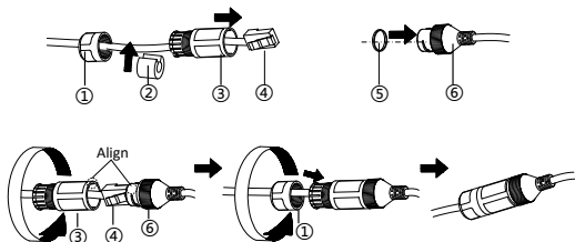
Рисунок 2-9 Установка гермовода
