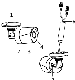
Рисунок 1-2 Цилиндрическая камера, Тип II (PoE)
