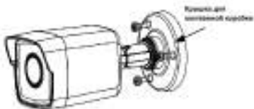
Рисунок 2-6 Крепление камеры на крышке для монтажной коробки
