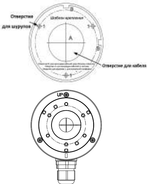
Рисунок 2-5 Шаблон крепления
