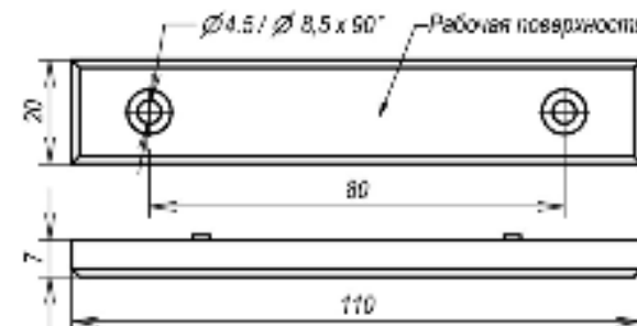
Рисунок 3 – Якорь
