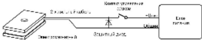
Рисунок 5 – Схема подключения замка
