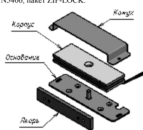
Рисунок 1 – Комплект поставки
